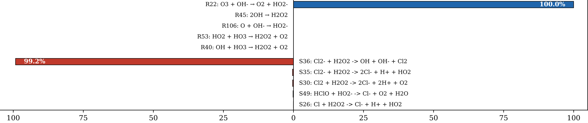
(d) H 2 O 2 (Σsrc = 4.63e-12 M/s)
